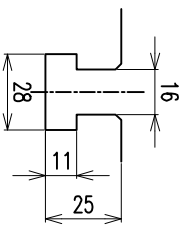
T-SLOT
