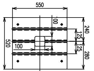
BOLSTER DIM.
