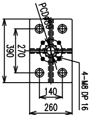
SLIDER DIM.
